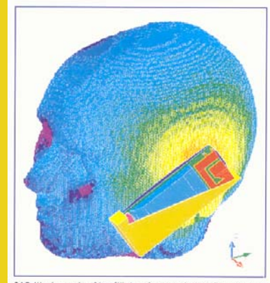
SAR-Werte an der Oberfläche eines Modellkopfes während eines Handytelefonats. Rot: SAR-Werte von circa 1 W/kg, Blau: SAR-Werte kleiner 0,002 W/kg (IMST GmbH, 2001)
